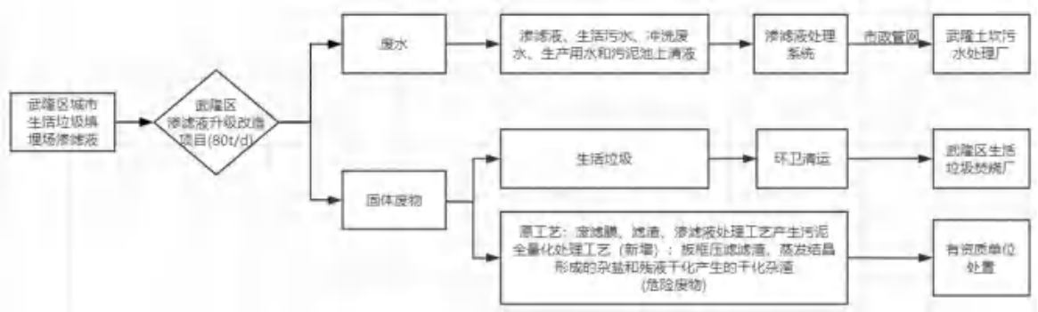
图2.5-2 武隆区城市生活垃圾填埋场渗滤液处理系统处理项目上下游设施关系图
