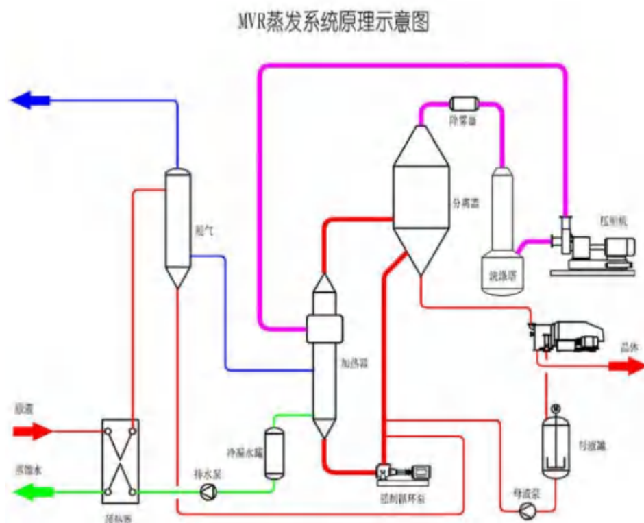
图3.3-2 MVR蒸发系统原理示意图
