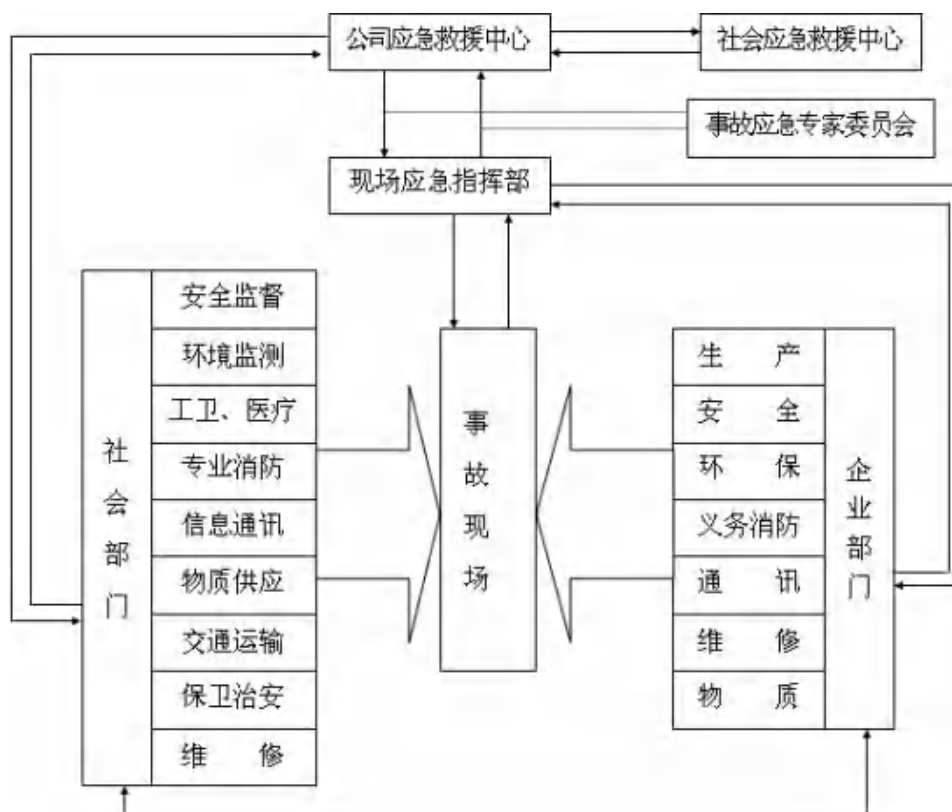
图9.1-2 风险事故应急组织系统基本框图
