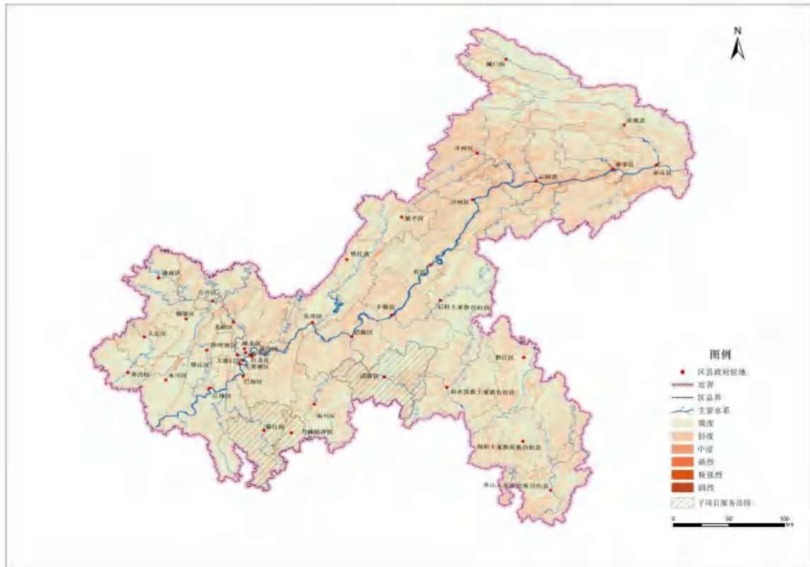
图4.2-2 项目位置及服务范围内土壤侵蚀现状图
